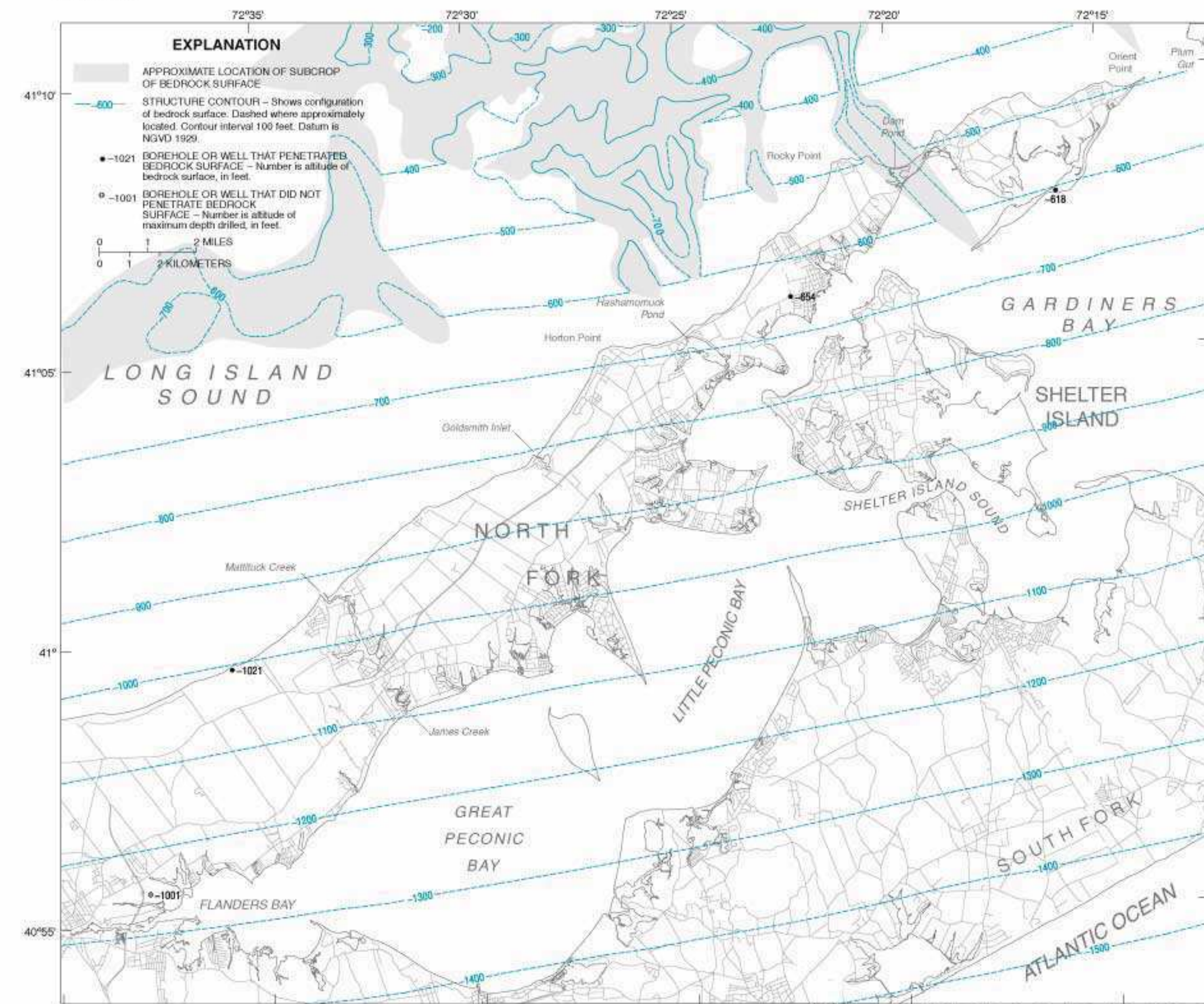
A. Bedrock
