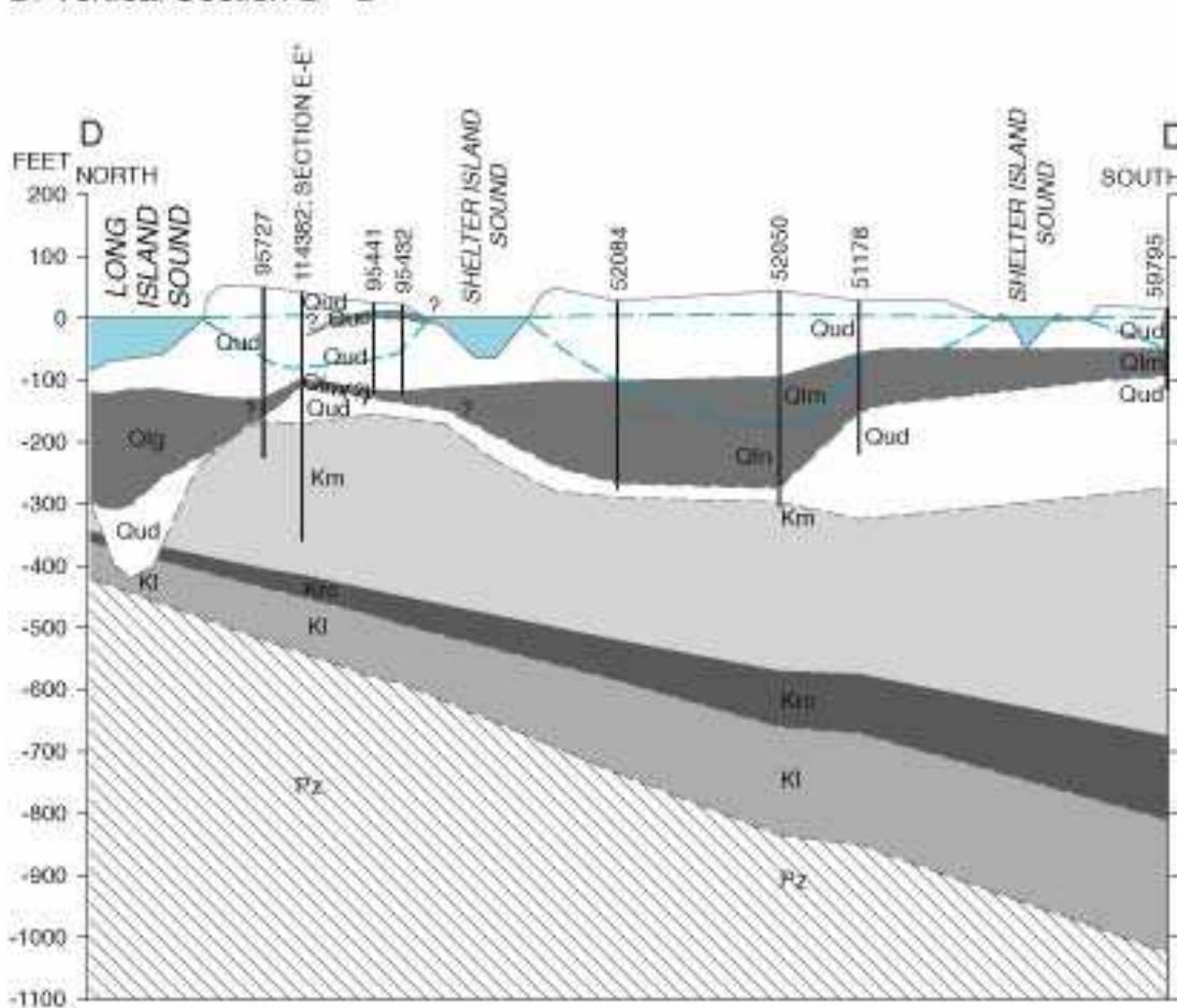
D. Vertical Section D - D'
